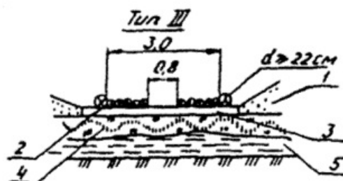
Графическая схема 2. Усиление ледовых переправ деревянным настилом: 1 - снеговой покров; 2 - колесопроды; 3 - поперечины; 4 - естественный ледяной покров; 5 - вода
